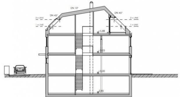
Schnitt
